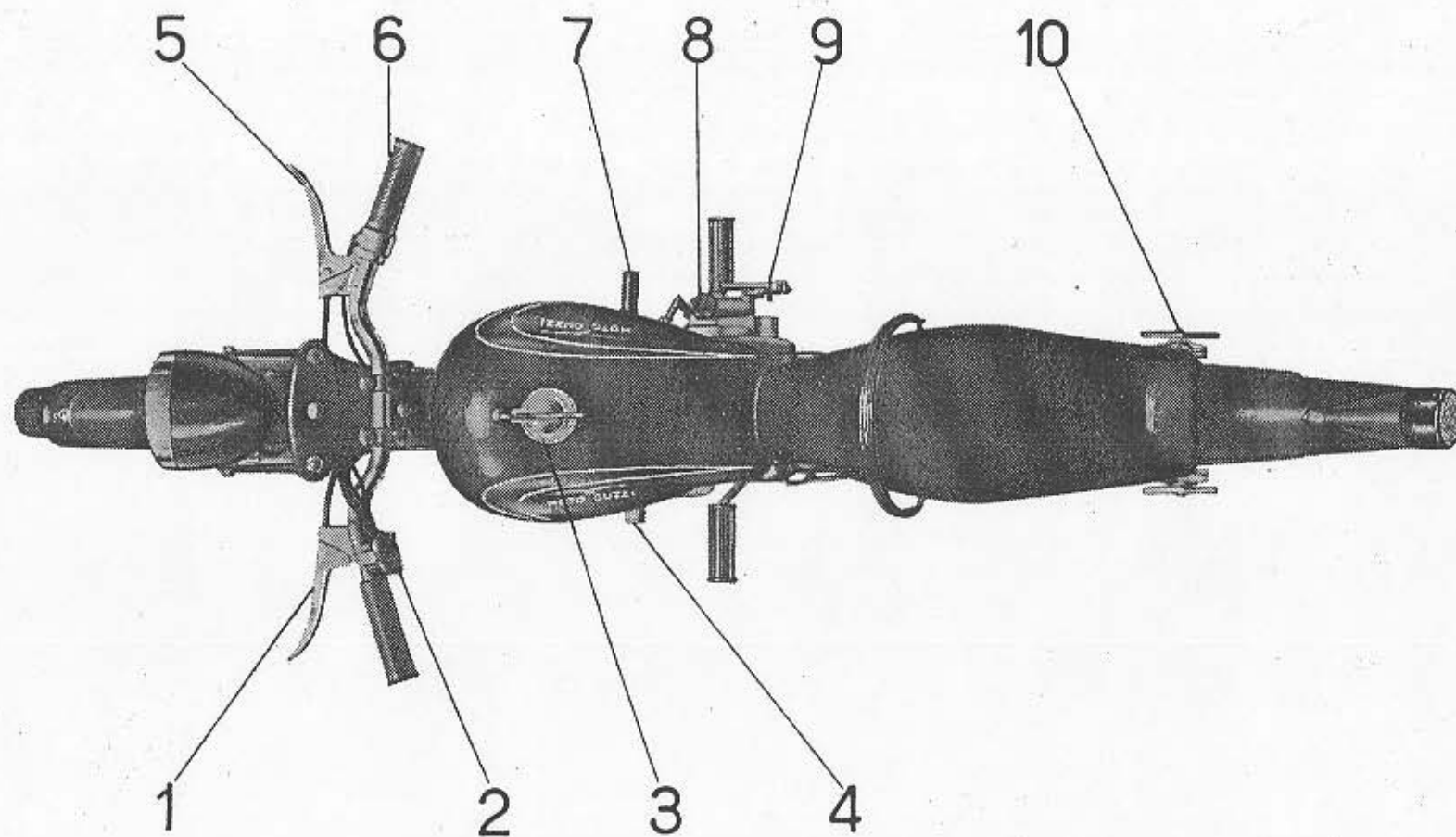
Fig. 2 - Comandi ed accessori
