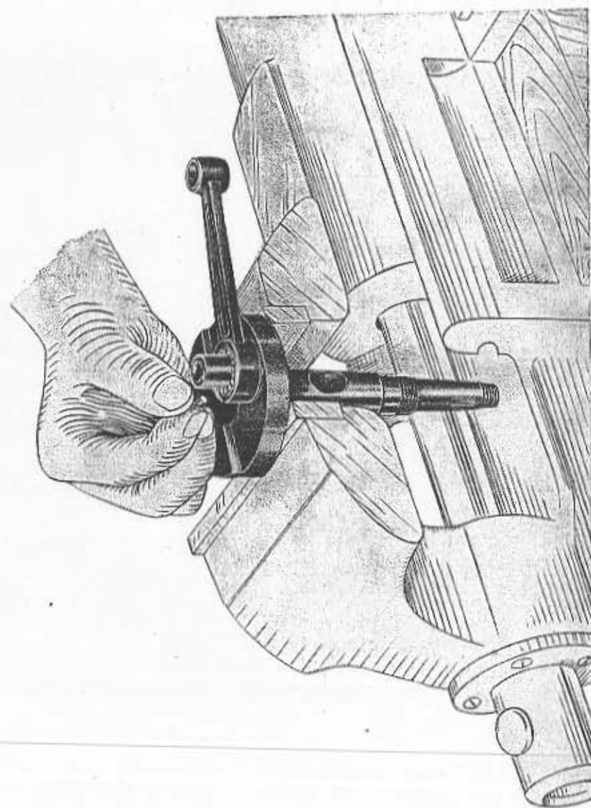
Fig. 18 - Montaggio dei rullini sull'albero a gomito
