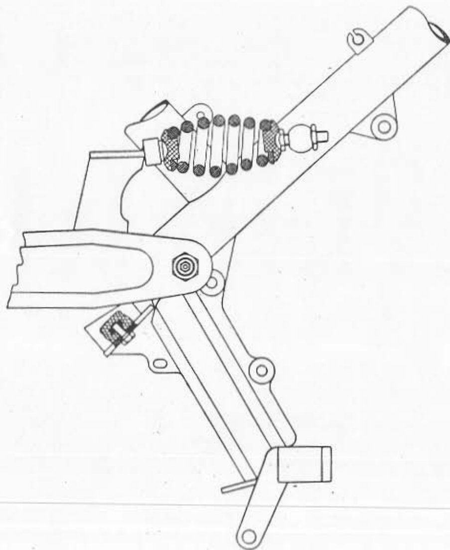
Fig. 24 - Molleggio posteriore
