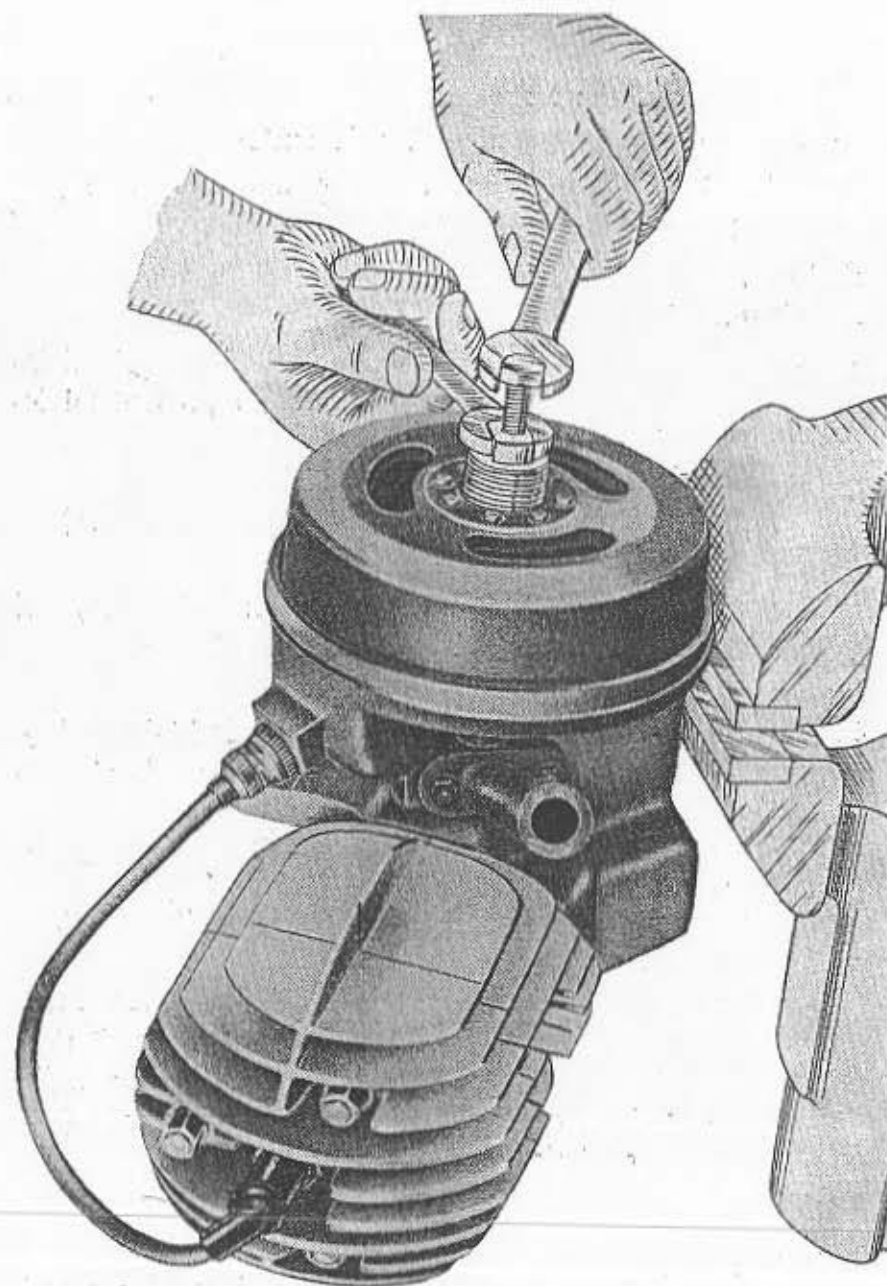
Fig. 11 - Come si toglie il volano magnete
