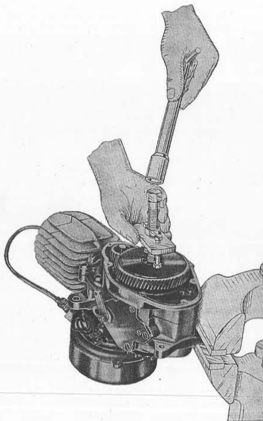
Fig. 8 - Come viene estratto il gruppo frizione
