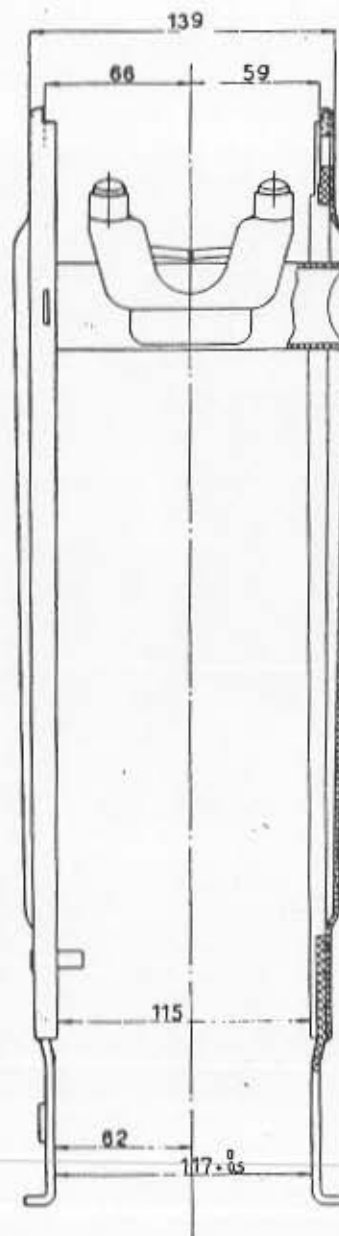
Fig. 25 - Forcellone oscillante
