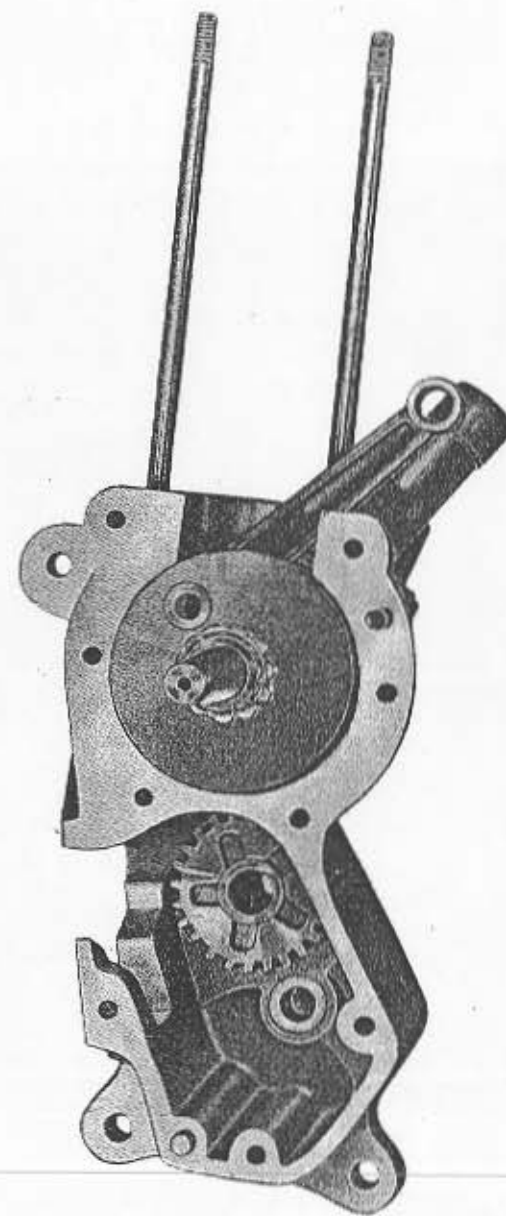
Fig. 13 - Come si trova il mezzo basamento sinistro, operata la separazione
