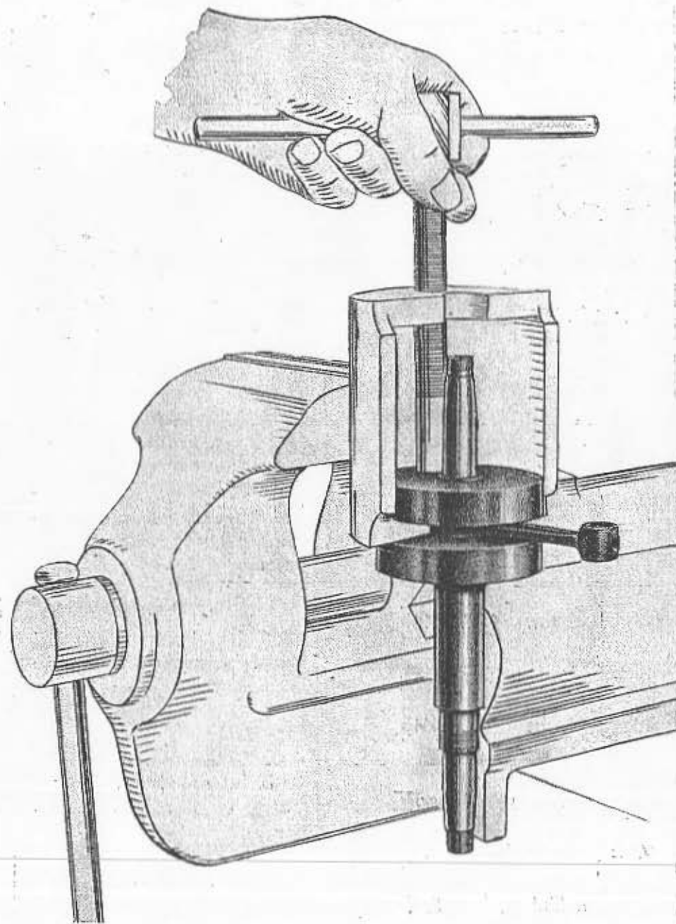
Fig. 17 - Come si estrae il perno per albero a gomito 27
