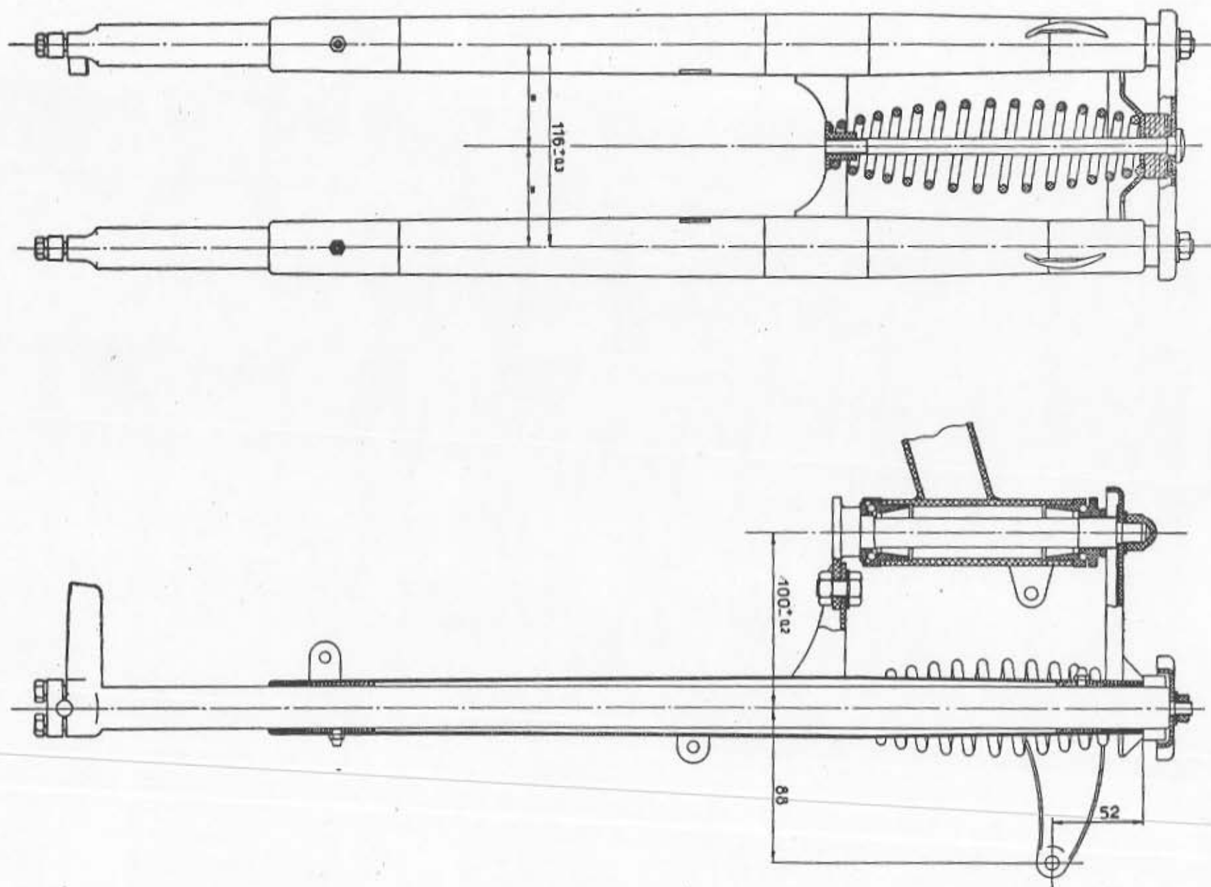
Fig. 22 - Forcella telescopica e sterzo
