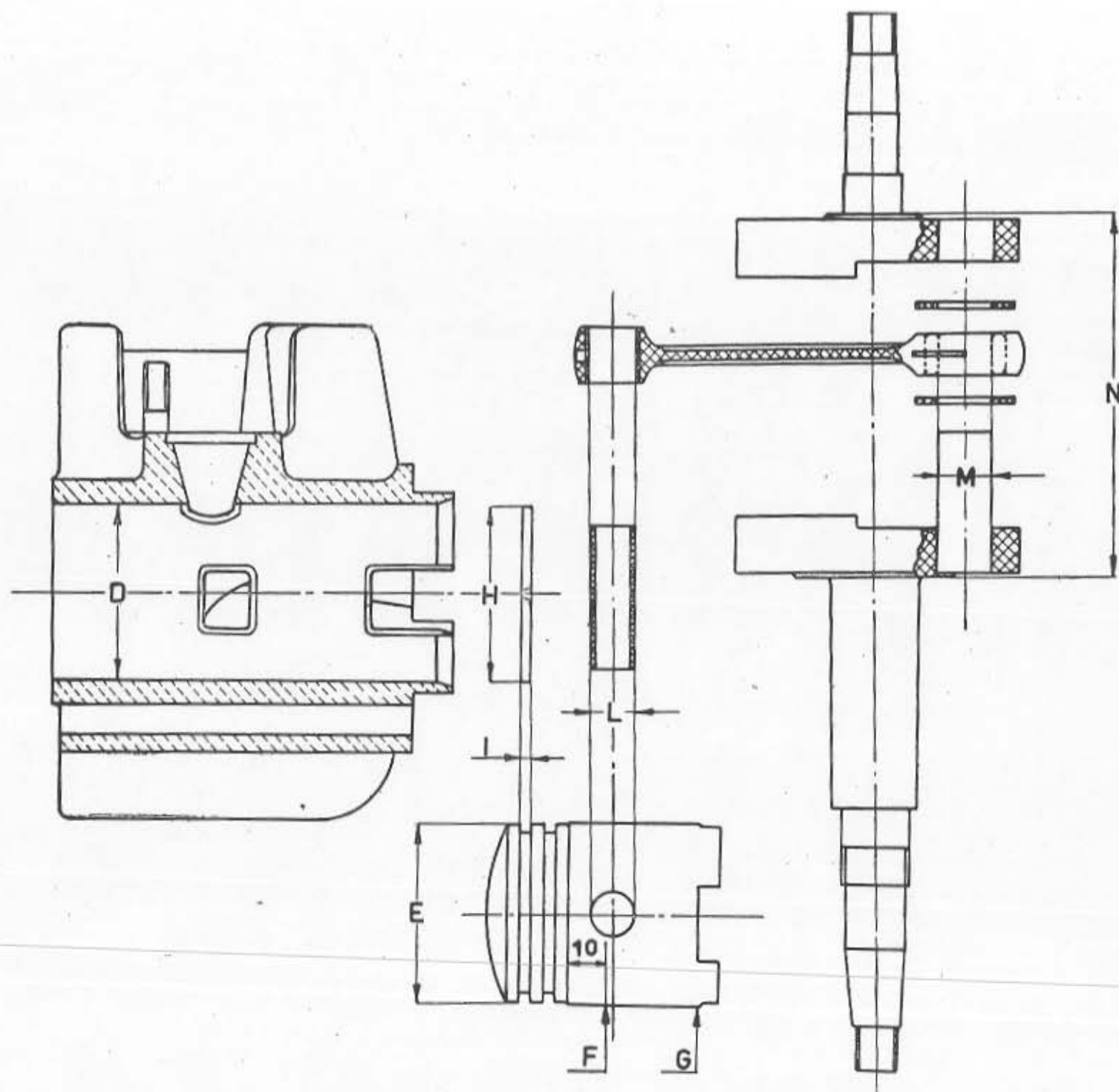
ORGANI DEL MANOVELLISMO
