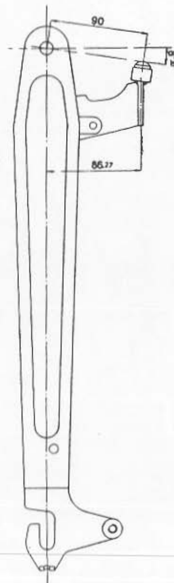
Fig. 25 - Forcellone oscillante
