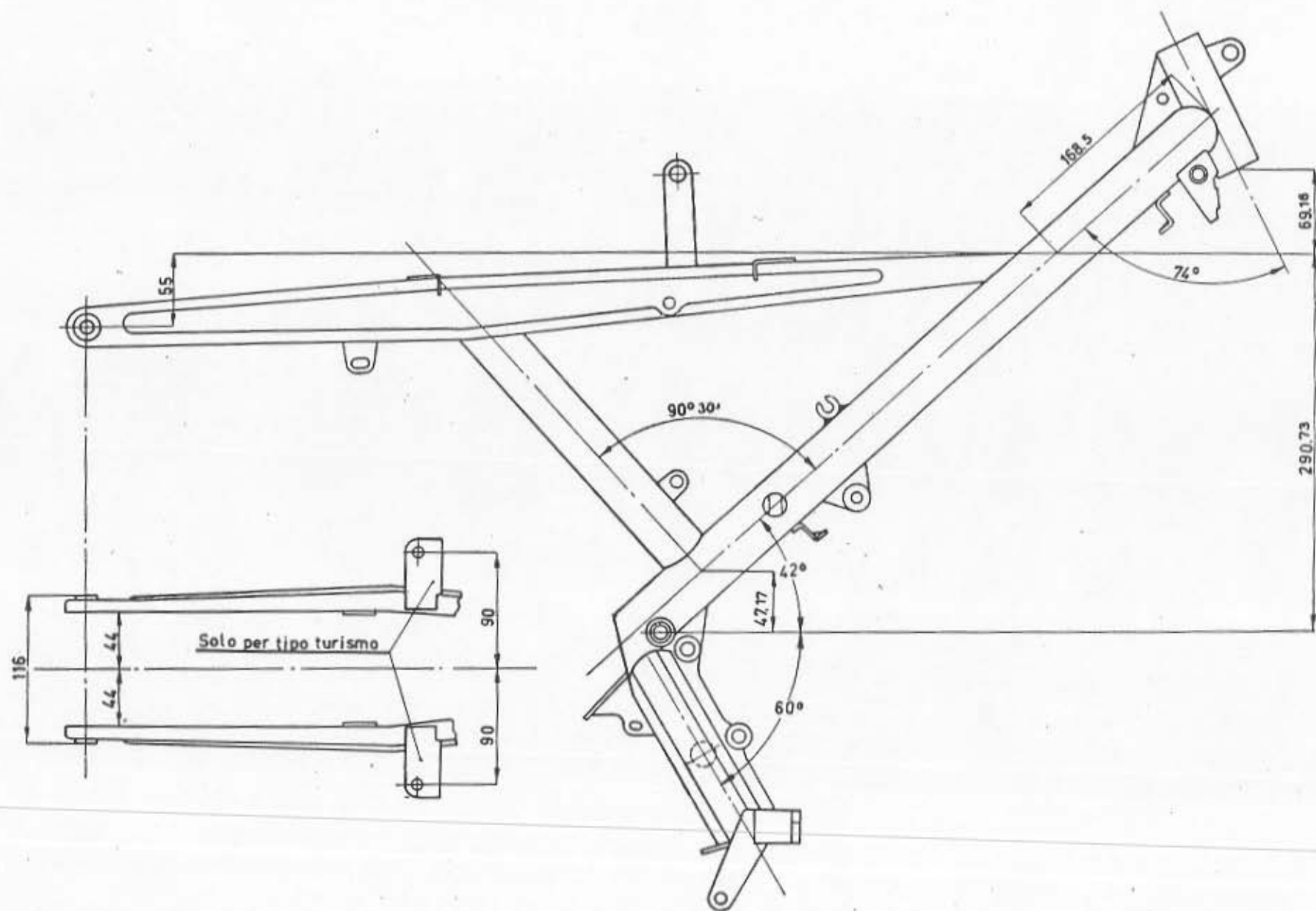
Fig. 23 - Telaio
