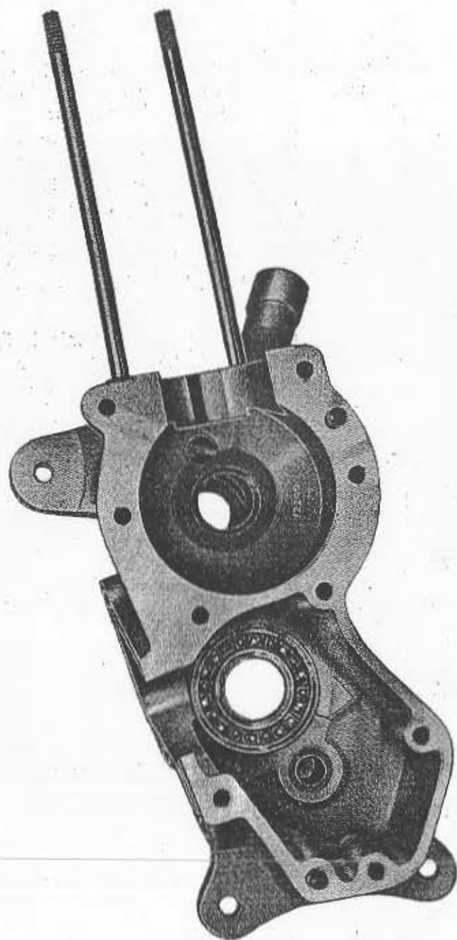
Fig. 16 - Mezzo basamento sinistro
