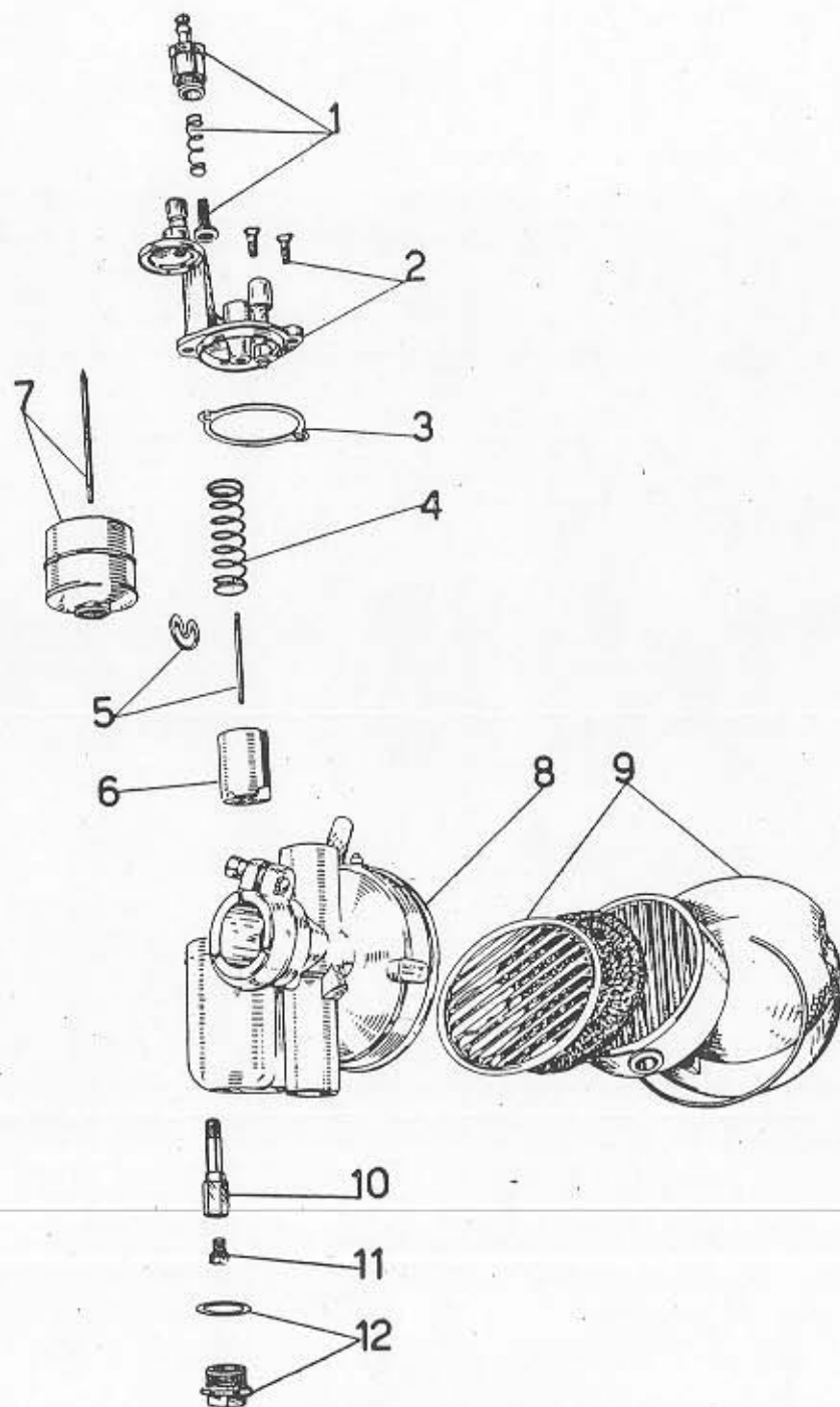
Fig. 19 bis - Carburatore smontato
